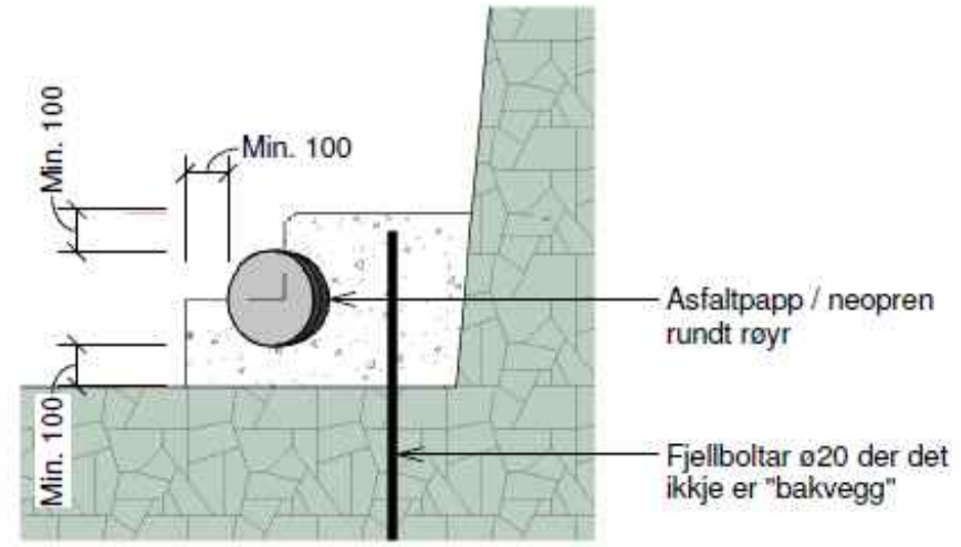
SNITT
