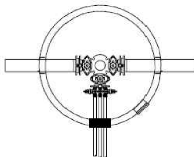
Løysing med koblingsflens
