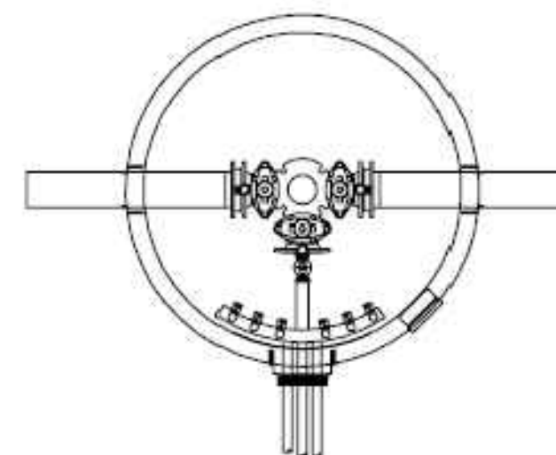
Løysing med manifold
