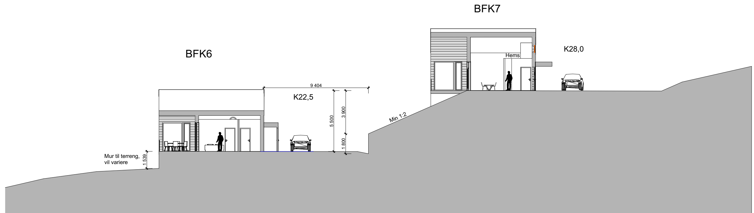
Snitt B
