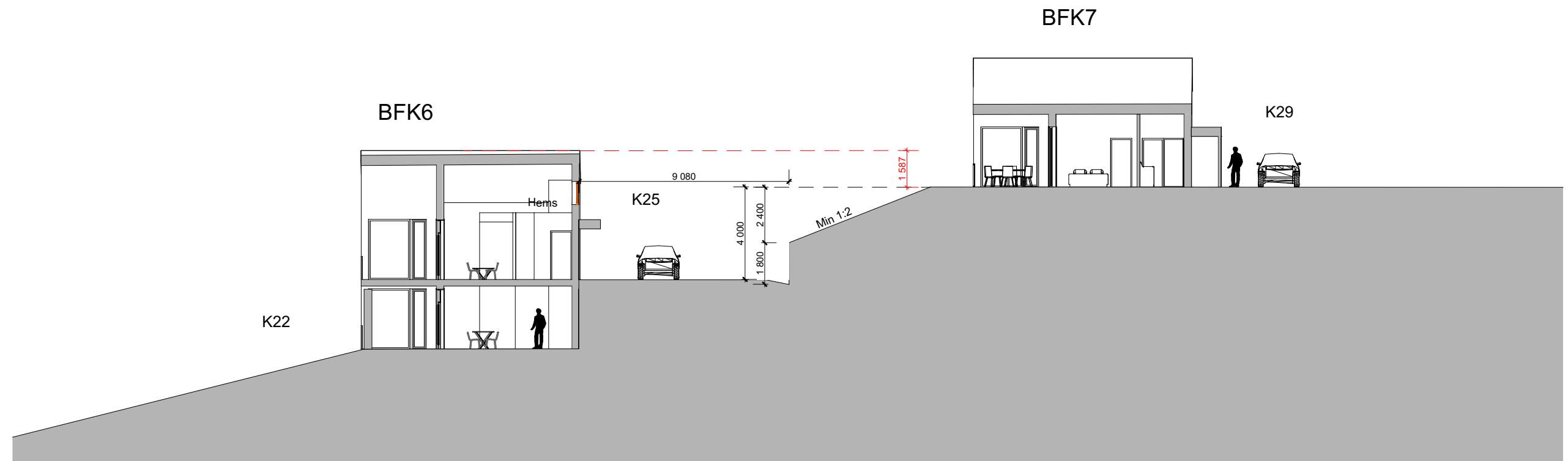
Snitt C
